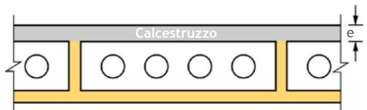
Solaio alveolare
