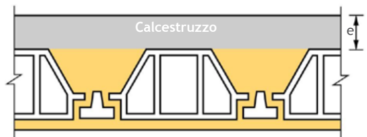
Solaio a travetti e blocchi
